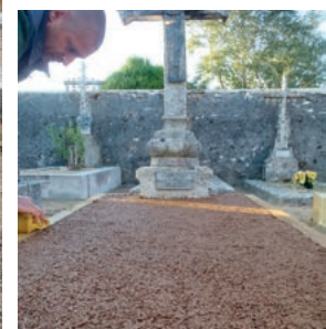
Mise en place du kit perméo
